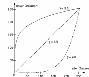
Gamma-Korrektur
