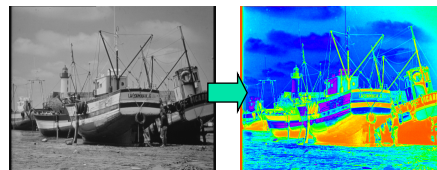
Graubild:
