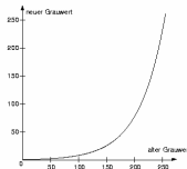
Exponential-Funktion
