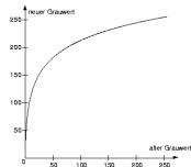
Logarithmus-Funktion
