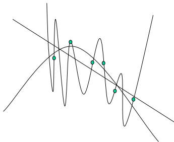
Kurvenapproximation an eine Menge von Punkten
