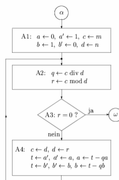
Abbildung 2: Ablaufdiagramm des erweiterten Euklid'schen Algorithmus
