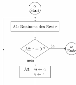
Abbildung 1: Ablaufdiagramm des Euklid'schen Algorithmus
